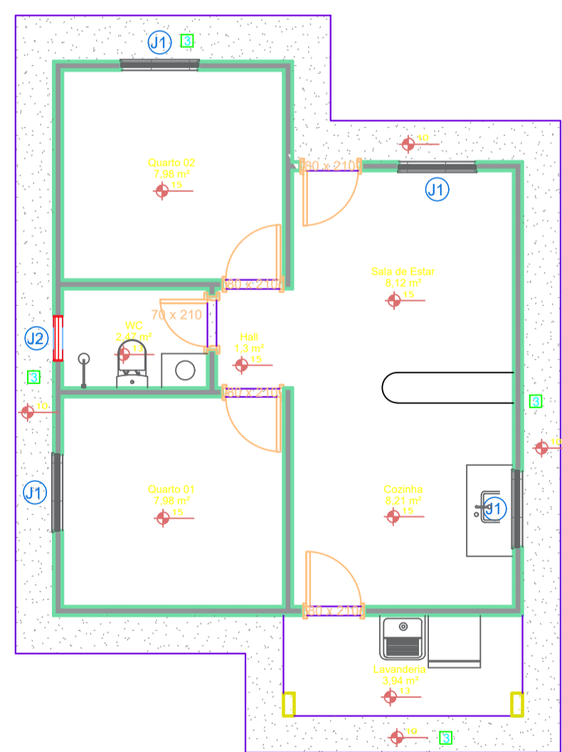
PLANTA BAIXA LAYOUT ESC.1:100
