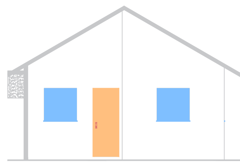
FACHADA NORTE ESC.1:100
